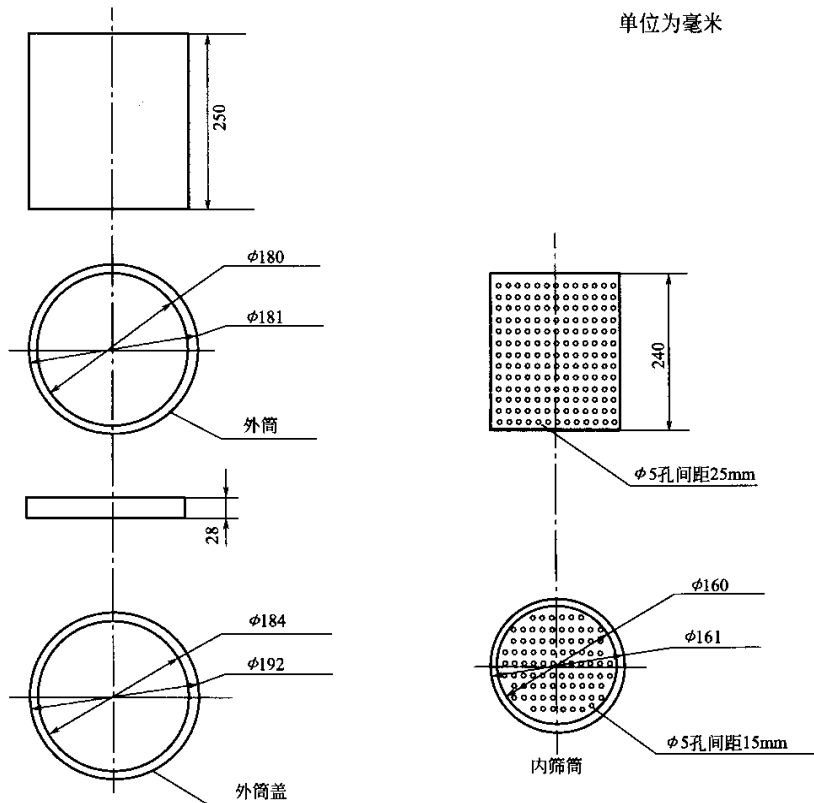
图 1 筛筒
